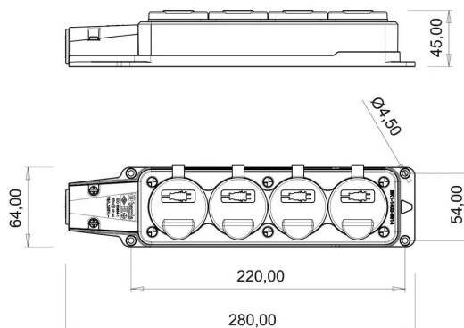
ГАБАРИТНЫЙ ЧЕРТЁЖ
