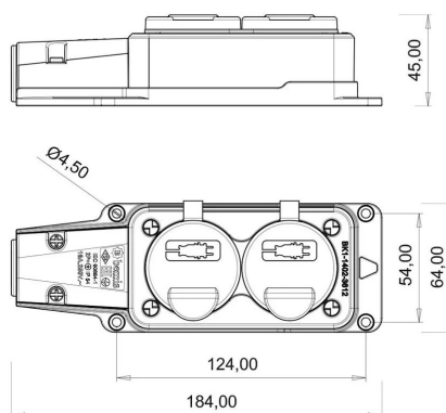
ГАБАРИТНЫЙ ЧЕРТЁЖ
