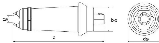
ГАБАРИТНЫЙ ЧЕРТЁЖ
