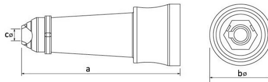
ГАБАРИТНЫЙ ЧЕРТЁЖ
