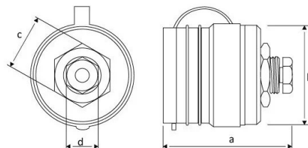
Ölçüler / Dimensions (mm)
