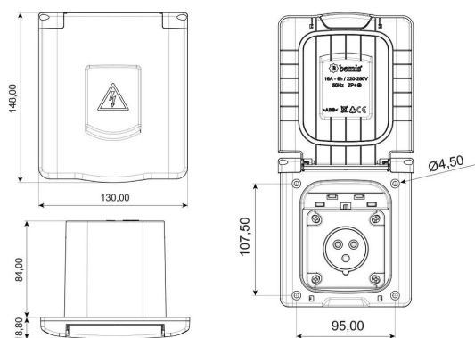
ГАБАРИТНЫЙ ЧЕРТЁЖ
