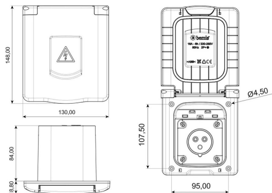
ГАБАРИТНЫЙ ЧЕРТЁЖ
