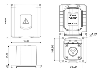
ГАБАРИТНЫЙ ЧЕРТЁЖ
