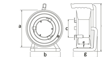
ГАБАРИТНЫЙ ЧЕРТЁЖ
