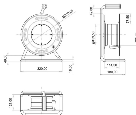
ГАБАРИТНЫЙ ЧЕРТЁЖ
