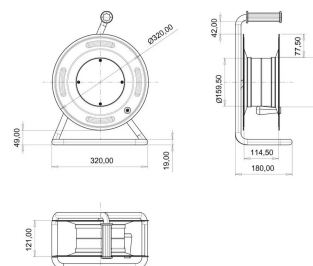
ГАБАРИТНЫЙ ЧЕРТЁЖ
