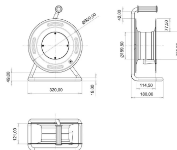
ГАБАРИТНЫЙ ЧЕРТЁЖ
