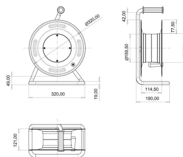
ГАБАРИТНЫЙ ЧЕРТЁЖ
