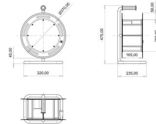
ГАБАРИТНЫЙ ЧЕРТЁЖ
