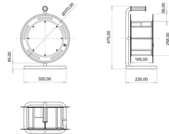
ГАБАРИТНЫЙ ЧЕРТЁЖ
