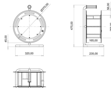
ГАБАРИТНЫЙ ЧЕРТЁЖ
