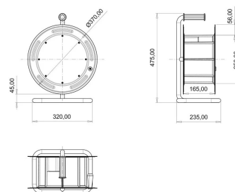
ГАБАРИТНЫЙ ЧЕРТЁЖ
