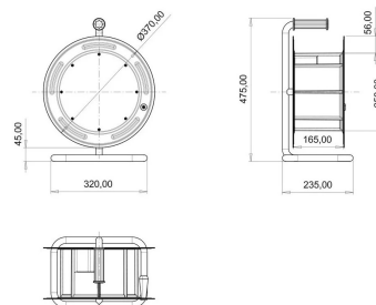
ГАБАРИТНЫЙ ЧЕРТЁЖ
