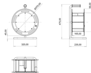
ГАБАРИТНЫЙ ЧЕРТЁЖ
