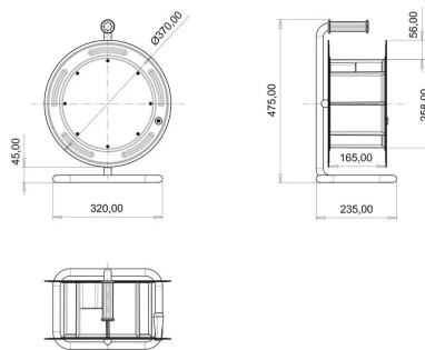
ГАБАРИТНЫЙ ЧЕРТЁЖ
