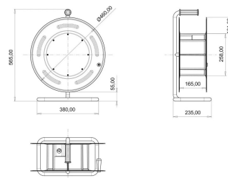
ГАБАРИТНЫЙ ЧЕРТЁЖ
