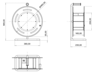
ГАБАРИТНЫЙ ЧЕРТЁЖ
