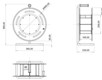
ГАБАРИТНЫЙ ЧЕРТЁЖ
