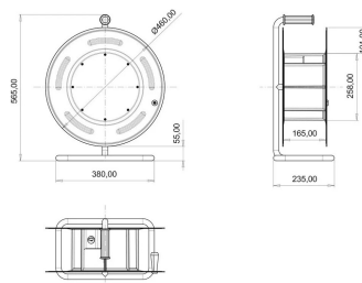
ГАБАРИТНЫЙ ЧЕРТЁЖ
