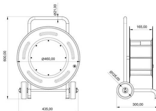
ГАБАРИТНЫЙ ЧЕРТЁЖ
