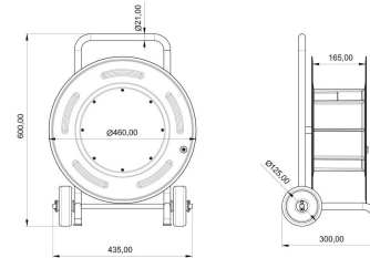
ГАБАРИТНЫЙ ЧЕРТЁЖ
