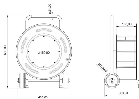
ГАБАРИТНЫЙ ЧЕРТЁЖ
