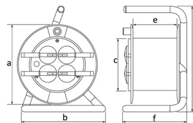
ГАБАРИТНЫЙ ЧЕРТЁЖ
