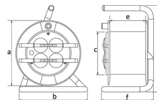
Ölçüler / Dimensions (mm)
