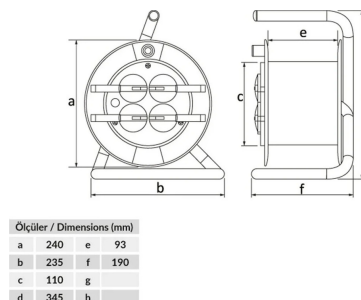
ГАБАРИТНЫЙ ЧЕРТЁЖ
