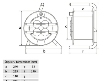
ГАБАРИТНЫЙ ЧЕРТЁЖ
