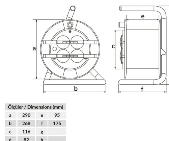
ГАБАРИТНЫЙ ЧЕРТЁЖ
