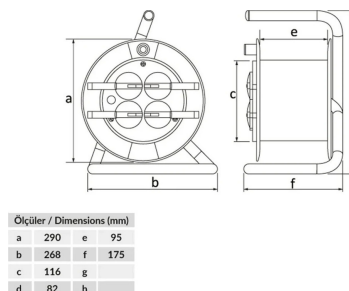
ГАБАРИТНЫЙ ЧЕРТЁЖ
