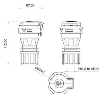
ГАБАРИТНЫЙ ЧЕРТЁЖ
