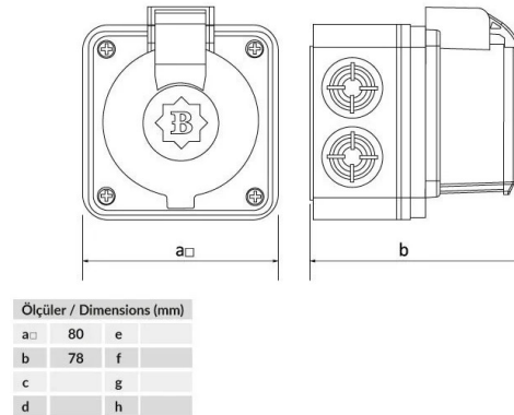
ГАБАРИТНЫЙ ЧЕРТЁЖ
