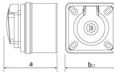
ГАБАРИТНЫЙ ЧЕРТЁЖ
