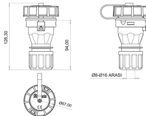
ГАБАРИТНЫЙ ЧЕРТЁЖ
