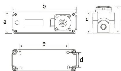
ГАБАРИТНЫЙ ЧЕРТЁЖ
