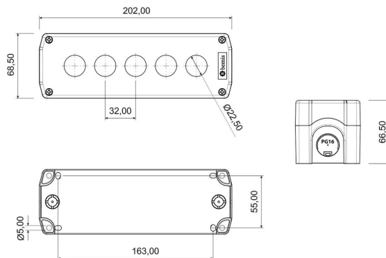
ГАБАРИТНЫЙ ЧЕРТЁЖ
