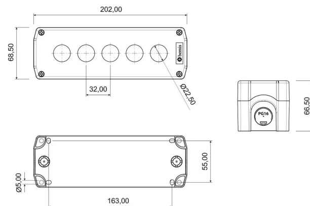
ГАБАРИТНЫЙ ЧЕРТЁЖ
