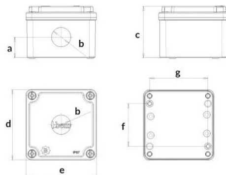
Ölçüler / Dimensions (mm)
