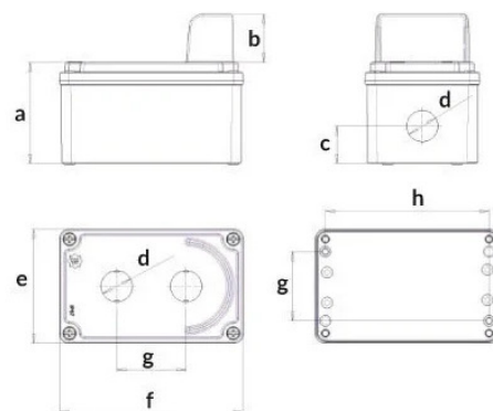
Ölçüler / Dimensions (mm)
