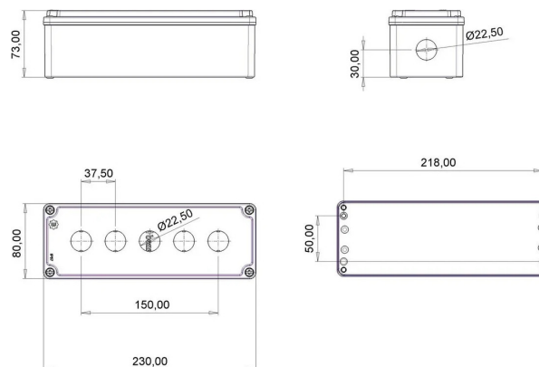
ГАБАРИТНЫЙ ЧЕРТЁЖ
