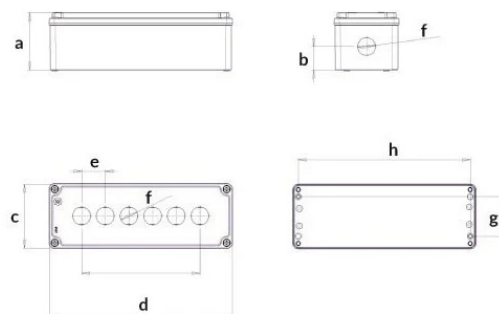
ГАБАРИТНЫЙ ЧЕРТЁЖ
