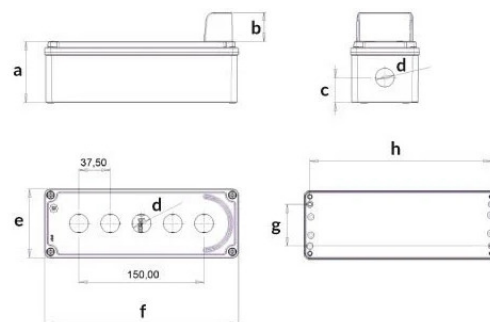
ГАБАРИТНЫЙ ЧЕРТЁЖ
