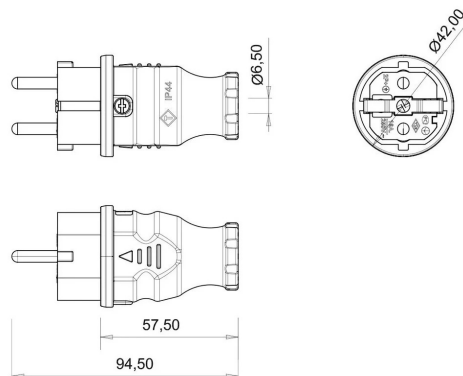
ГАБАРИТНЫЙ ЧЕРТЁЖ
