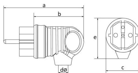
ГАБАРИТНЫЙ ЧЕРТЁЖ
