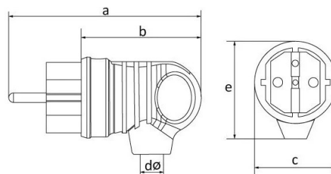
ГАБАРИТНЫЙ ЧЕРТЁЖ
