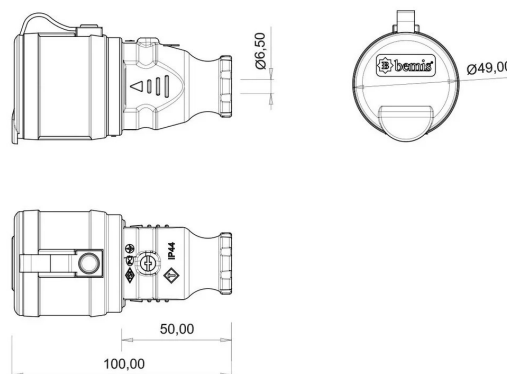
ГАБАРИТНЫЙ ЧЕРТЁЖ
