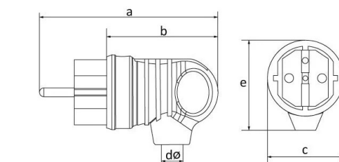
ГАБАРИТНЫЙ ЧЕРТЁЖ
